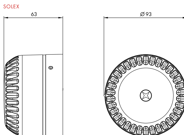
Höhe mit Deep Base | Height with Deep Base = 91mm Höhe mit U-Base | Height with U-Base = 94mm
