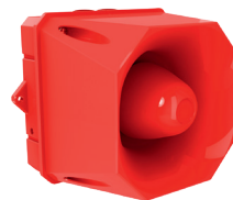
X10 MINI akustischer Signalgeber · IP66 & IP69K · max. 100 dB (A)
