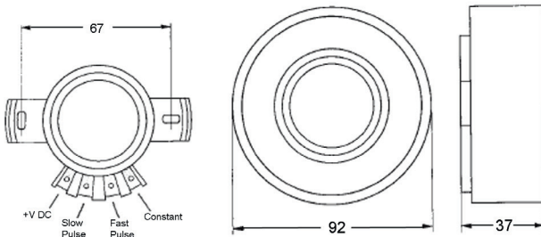
Sirenen-Unterteil mit Reflektorring
